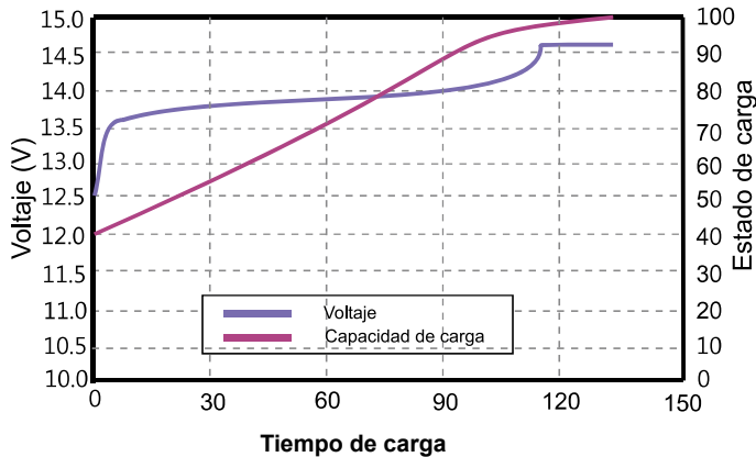
Curva de estado de carga ©0,50 25°C
