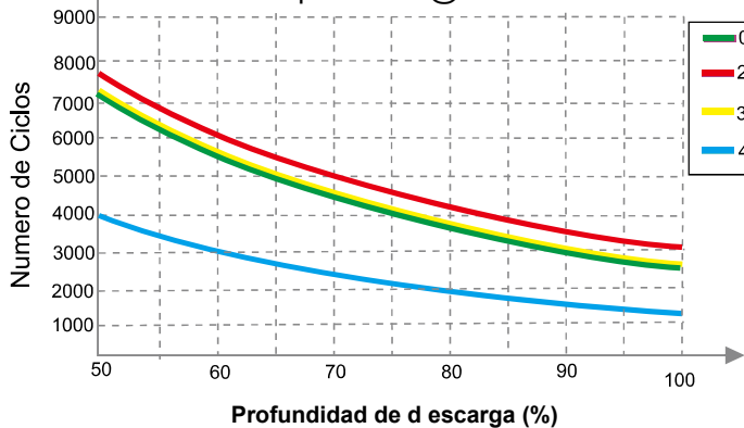
Curva de vida de diferentes DOD y ciclos de diferentes temperaturas @0.2C
